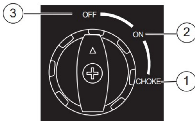
Малюнок 3-2. Позиції ВИМК/УВИМК/ДРОСЕЛЬ
